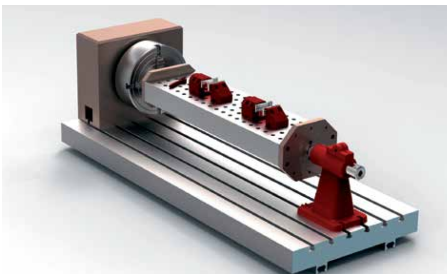
Modélisation réalisée avec la CAO 3D SpaceClaim distribuée par MW Programmation.
