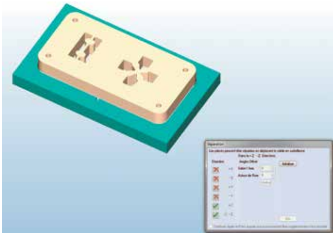
Gestion d'une machine à électro-érosion à fil avec le logiciel Visi Wire.
